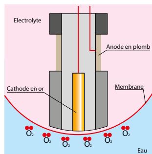
Intérieur d'une sonde oxygène (grossissement)
